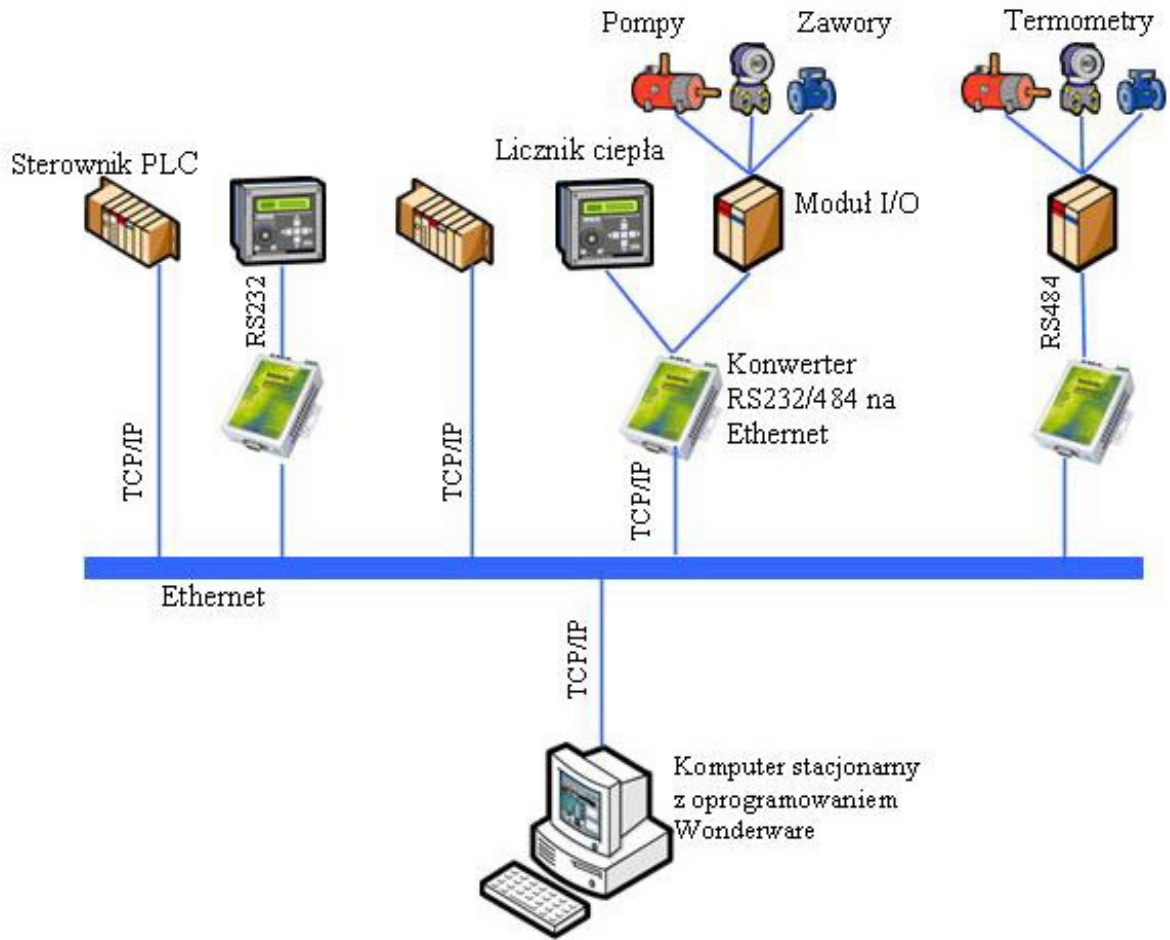
Poglądowy schemat systemu
