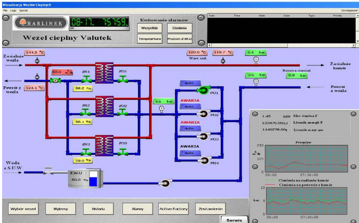
Okno główne aplikacji wizualizacyjnej
